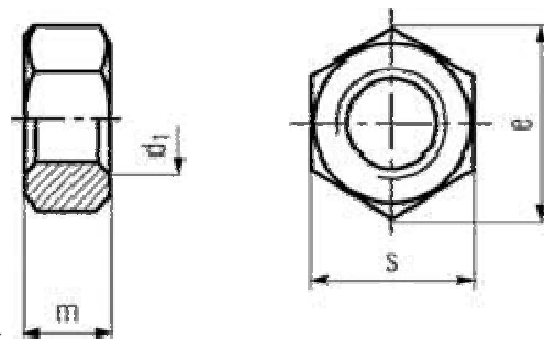
DIN 934 - Гайка шестостенна
